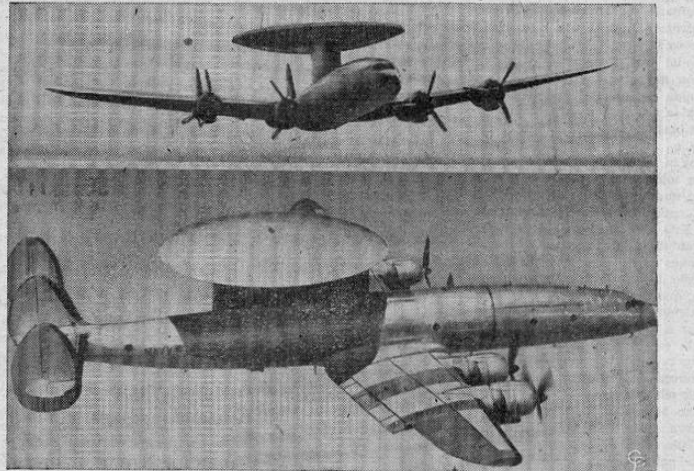
He aquí dos vistas del avión de estudios de radar de la marina de guerra norteamericana apodado "Platillo Volador" en vuelo sobre South Weymouth, Massachusetts. El avión Lockheed es capaz de captar la presencia de aviones de bombardeo enemigos desde los bordes del espacio hasta la superficie de la tierra. El extraño avión parece como un "platillo volador" a caballo sobre un aeroplano. La gran cúpula redonda de radar aloja la antena para un ojo electrónico de supervisión que permite realizar el trabajo de docenas de estaciones de radar de tierra. El gran disco tiene aproximadamente 37 pies de diámetro. (INP).
